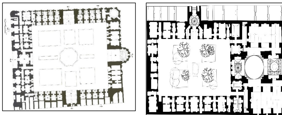
ب. پلان مدرسه حاج صفرعلی
