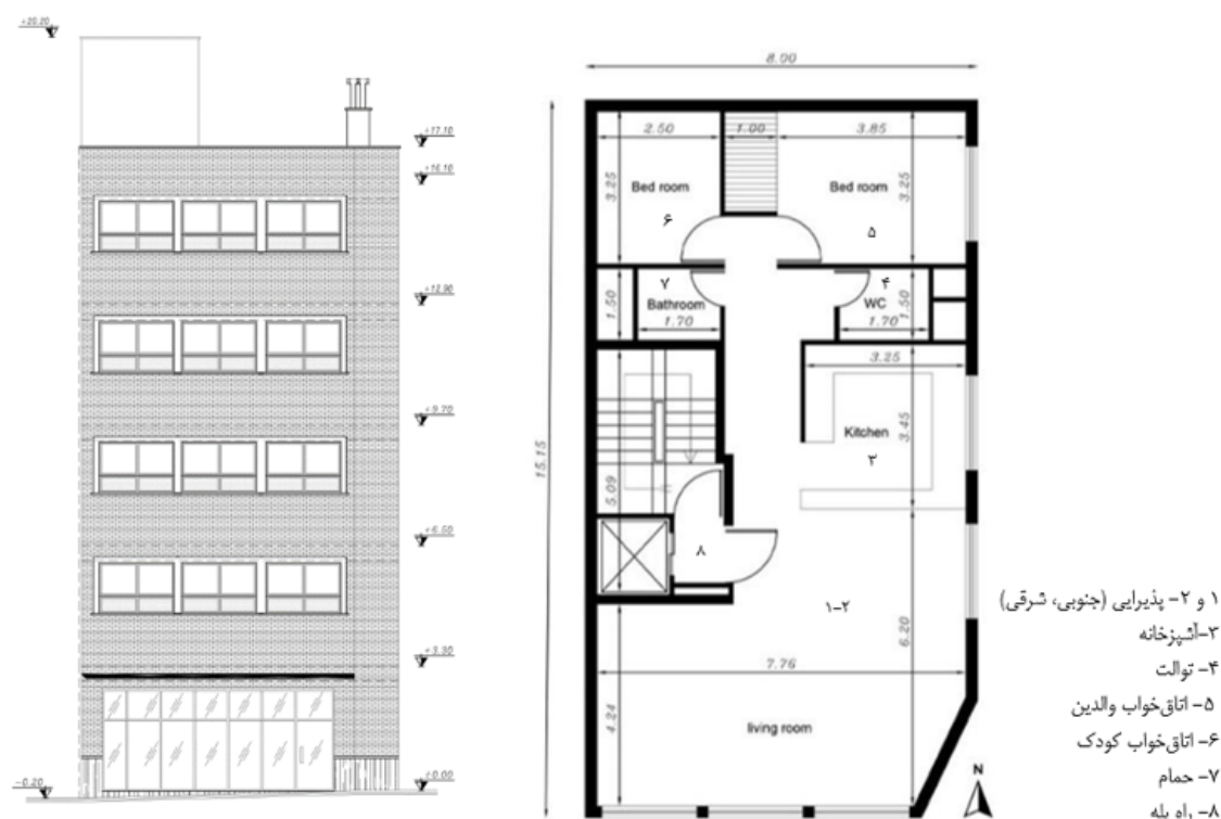
شکل ۱: سمت راست: پلان طبقه پنجم و مشخصات فضاهای مورد بررسی، سمت چپ: نمای اصلی ساختمان (منبع: نگارندگان) Fig 1: Right: the plan of the fifth floor and the characteristics of the investigated spaces, Left: the main view of the building
